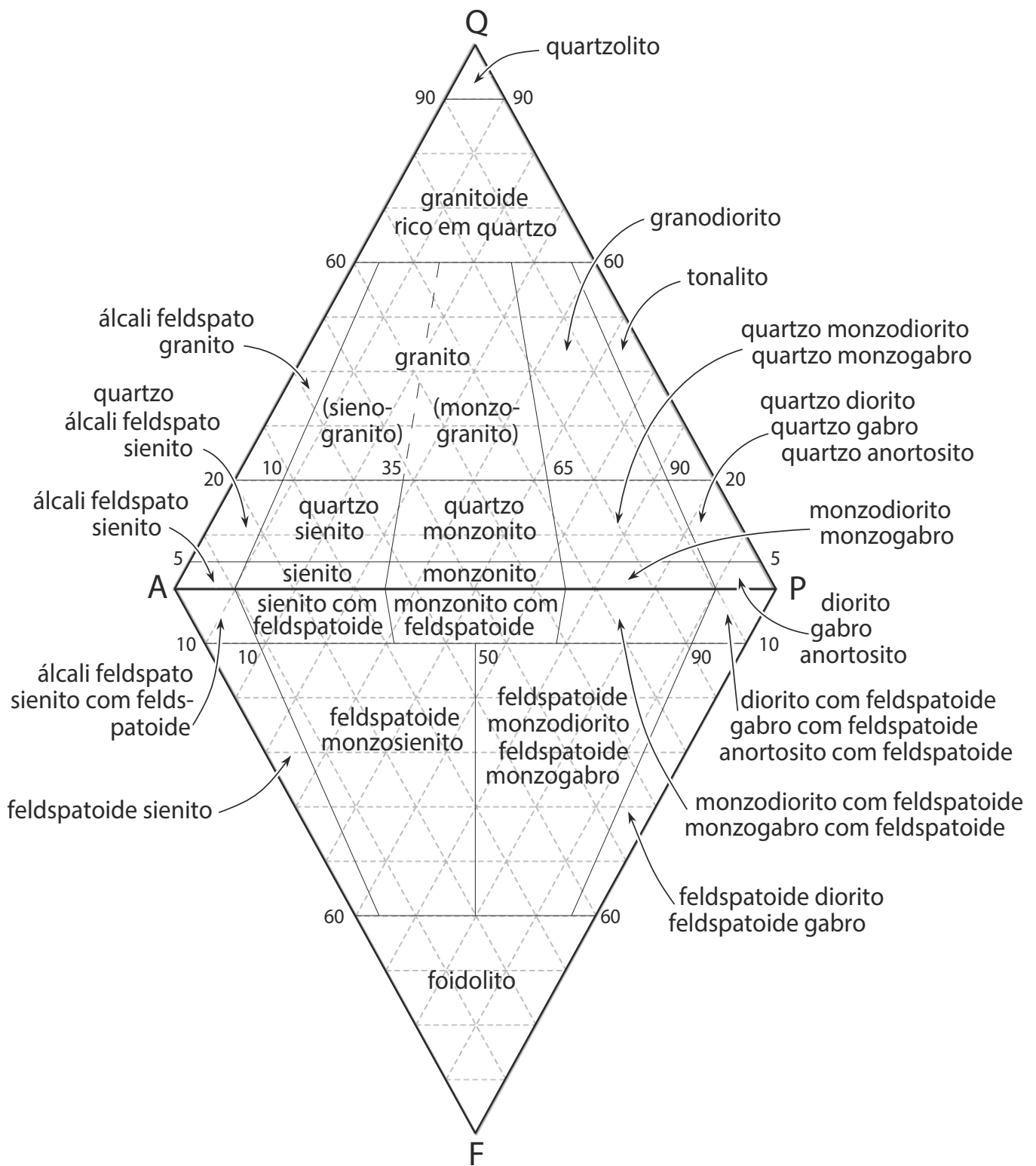
Diagrama QAPF para classificação modal de rochas plutônicas ( baseado em Streckeisen, 1976). Os extremos do losango são: Q = quartzo, A = Feldspato alcalino, P = plagioclásio e F = feldspatoídes. Este diagrama não deve ser usado para rochas cujo o conteúdo de minerais máficos, M, é maior que 90%.
