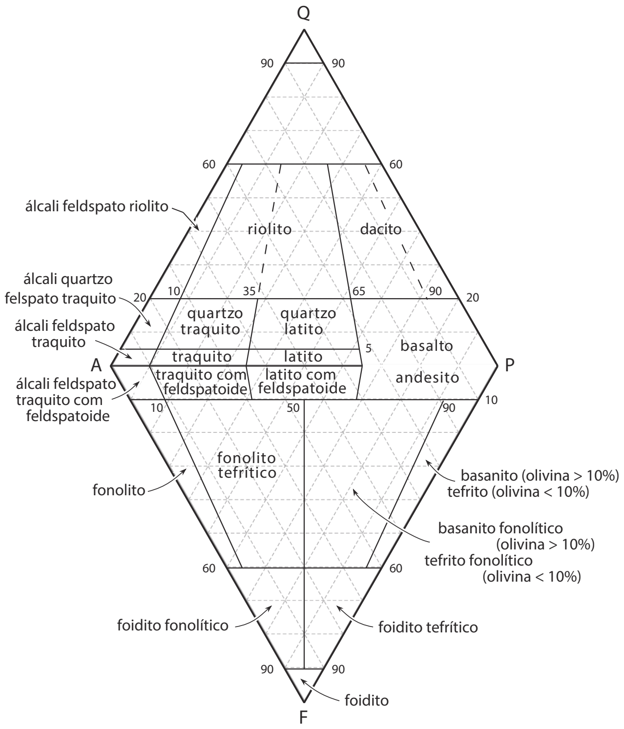
Diagrama QAPF para classificação modal de rochas vulcânicas (baseado em Streckeisen, 1978). Os extremos do losango são: Q = quartzo, A = feldspato alcalino, P = plagioclasio e F = feldspatoide. Este diagrama não deve ser usado para rochas com conteúdo de minerais máficos, M, maiores que 90%.
