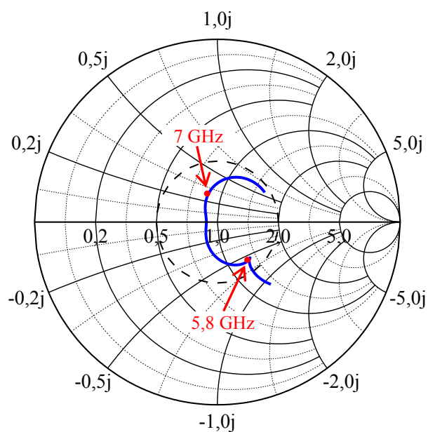
Figura 69 – Impedância de entrada otimizada na carta de Smith para a antenna.
