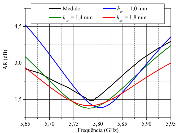
Figura 126 – Variação da AR da antena na banda inferior em função da camada de ar.
