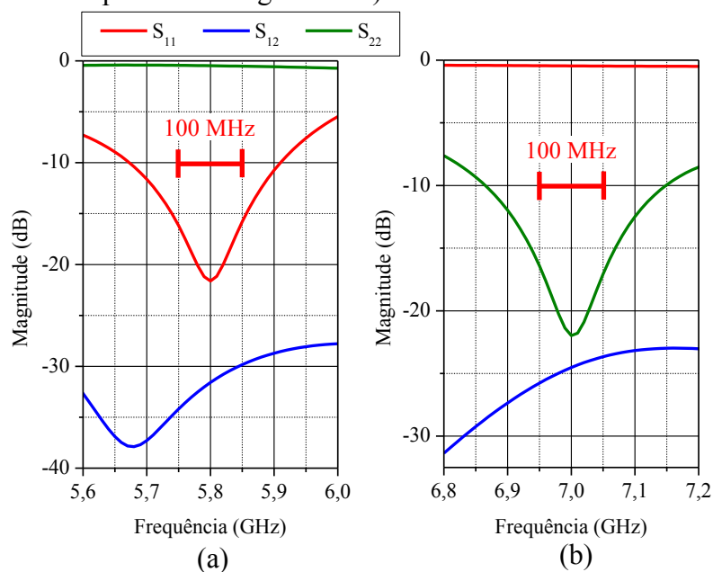
Figura 117 – Parâmetros S finais da antena nas faixas de operação (as curvas de S_{12} e S_{21} são coincidentes devido à reciprocidade da geometria).
