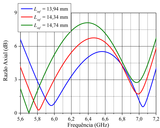
Figura 62 – Variação da razão axial em função de L_{inf} .
