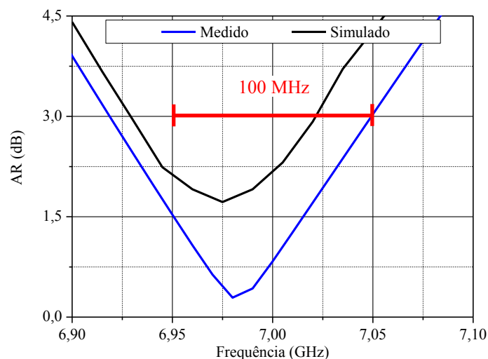
Figura 125 – Curvas de razão axial medida e simulada na banda superior da antena.
