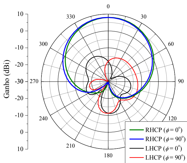
Figura 53 – Diagrama de ganho em 5,8 GHz.
