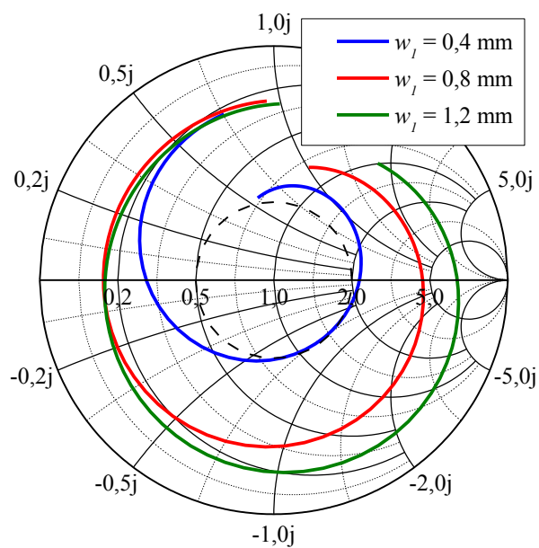
Figura 34 – Variação da impedância de entrada na carta de Smith para a banda superior em função de w_I .
