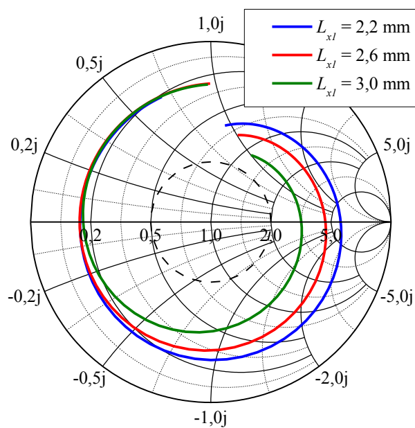
Figura 37 – Variação da impedância de entrada na carta de Smith para a banda superior em função de L_{xl} .
