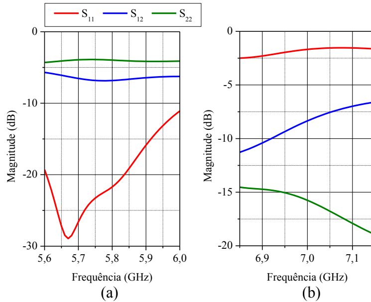
Figura 82 – Parâmetros S da antenna (as curvas de S_{12} e S_{21} são coincidentes devido à reciprocidade da geometria).
