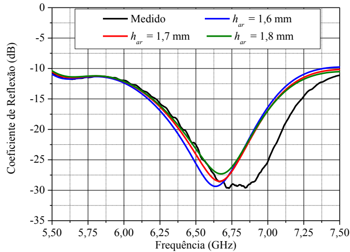
Figura 78 – Efeito da altura da camada de ar no coeficiente de reflexão.
