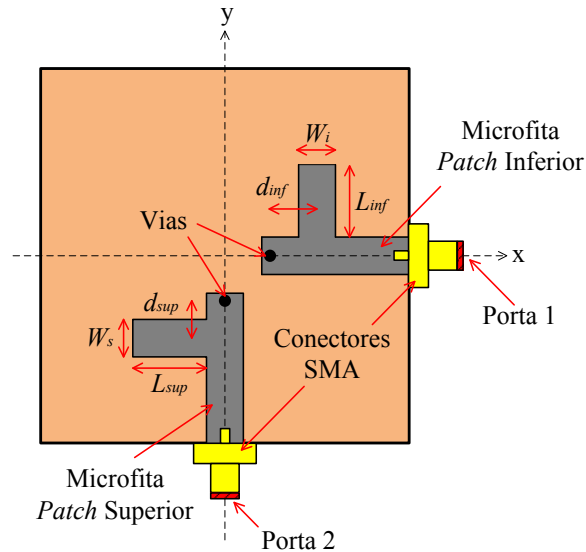
Figura 80 – Detalhamento do sistema de alimentação da antena.
