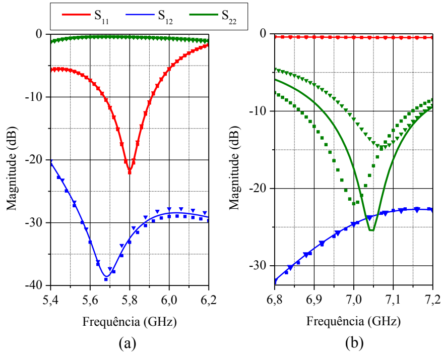
Figura 105 – Análise paramétrica dos parâmetros S da antena nas duas bandas de operação (as curvas de S_{12} e S_{21} são coincidentes devido à reciprocidade da geometria).
