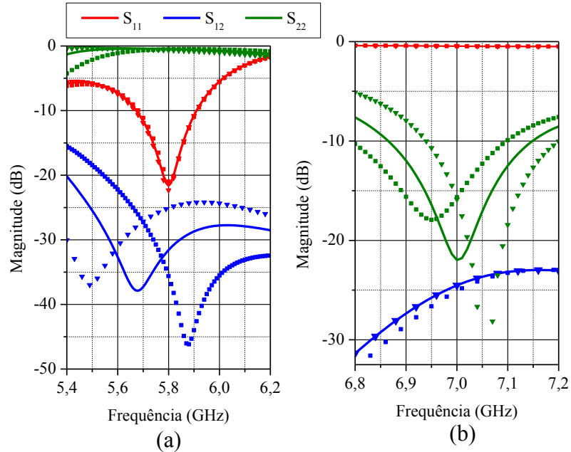
Figura 115 – Análise paramétrica dos parâmetros S da antenna nas duas bandas de operação (as curvas de S_{12} e S_{21} são coincidentes devido à reciprocidade da geometria).
