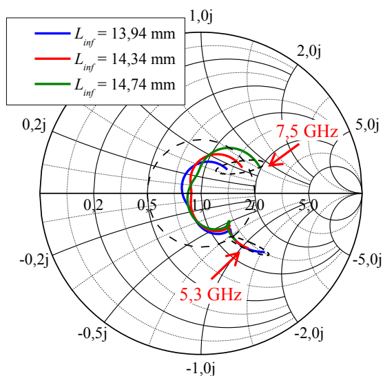
Figura 63 – Variação da impedância de entrada na carta de Smith em função de L_{inf} .
