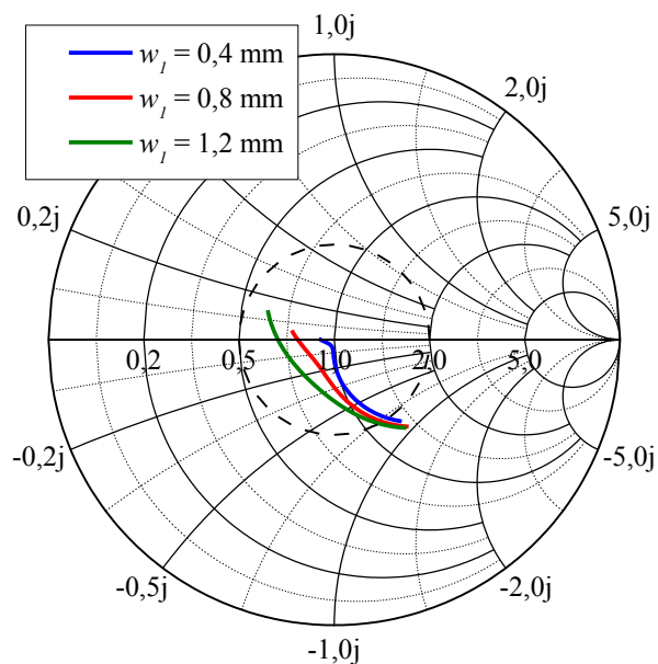
Figura 33 – Variação da impedância de entrada na carta de Smith para a banda inferior em função de w_I .
