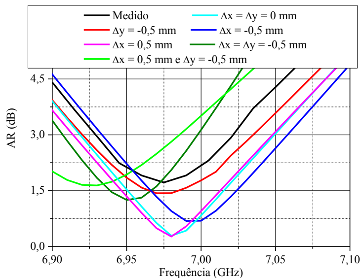
Figura 128 – Variação da AR da antenna na banda superior em função dos desalinhamentos entre os laminados.
