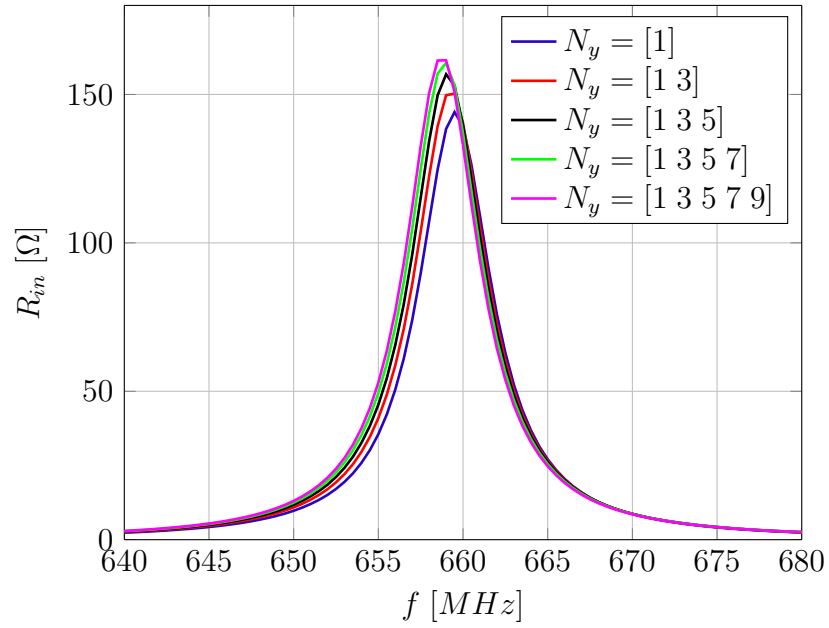
Figura 16 – Convergência da resistência de entrada para diferentes números de modos na direção de y .
