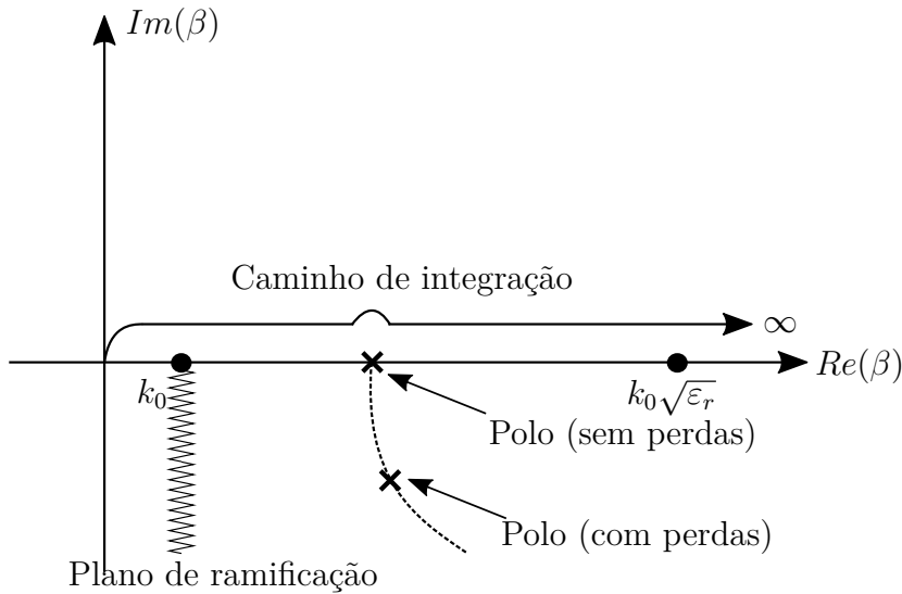
Figura 7 – Caminho de integração no plano complexo \beta e local geométrico do polo em função da perda dielétrica.
