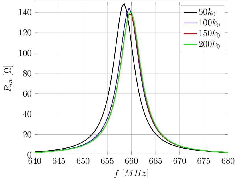
Figura 14 – Convergência da resistência de entrada para a variação do limite do caminho de integração.
