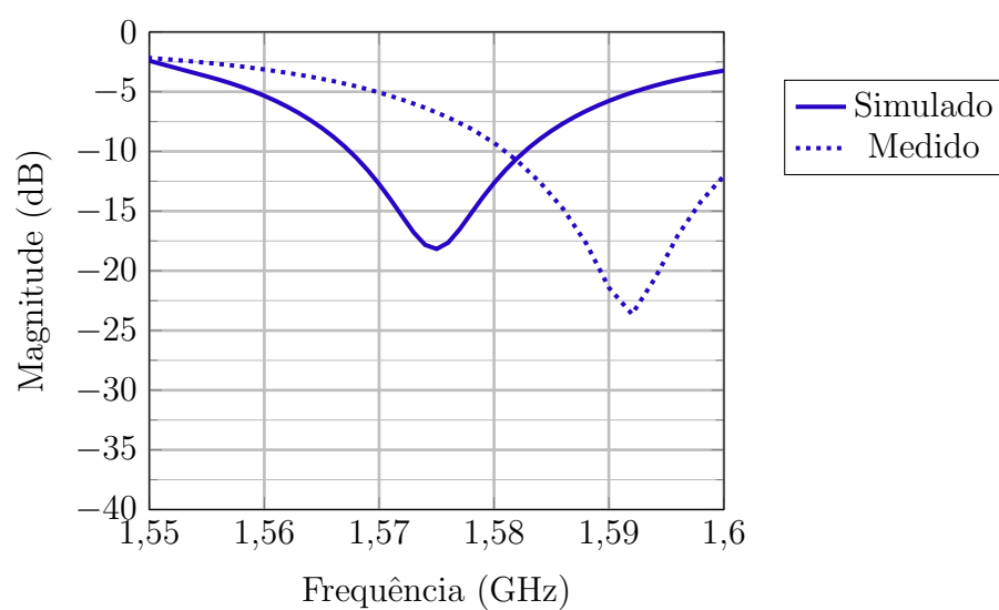
Figura 114 – Comparação entre os coeficientes de reflexão em função da frequência para a antena projetada em Banda L considerando \varepsilon_r = 12 .
