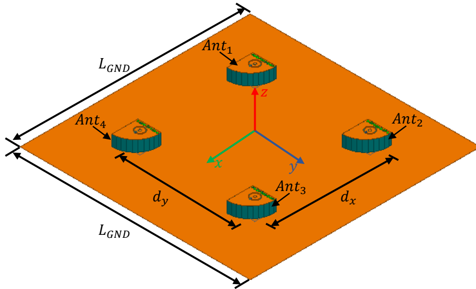
Figura 42 – Rede 2 \times 2 em Banda S.
