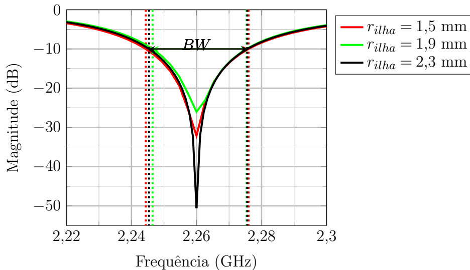
Figura 38 – Coeficientes de reflexão em função da frequência para diferentes tamanhos de ilha.
