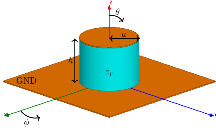
Figura 19 – Antena dielétrica ressoadora cilíndrica com carregamento metálico.
