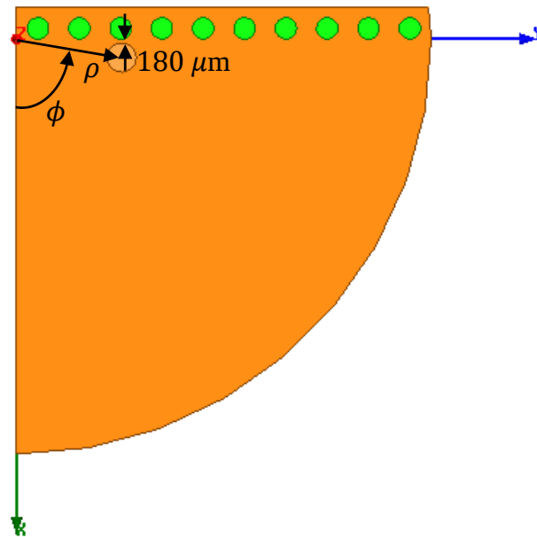
Figura 87 – Vista superior do posicionamento da ponta de prova coaxial em \rho = 5 \text{ mm} e \phi = 80^\circ .
