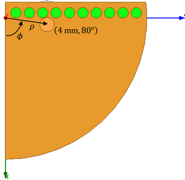
Figura 30 – Vista superior do posicionamento da ponta de prova coaxial em \rho = 4 mm e \phi = 80^\circ .
