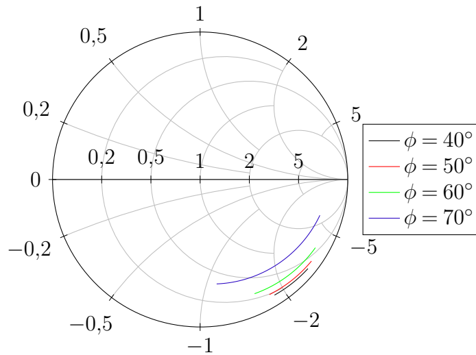
Figura 33 – Análise da impedância de entrada com a ponta de prova coaxial em \rho = 8 mm.
