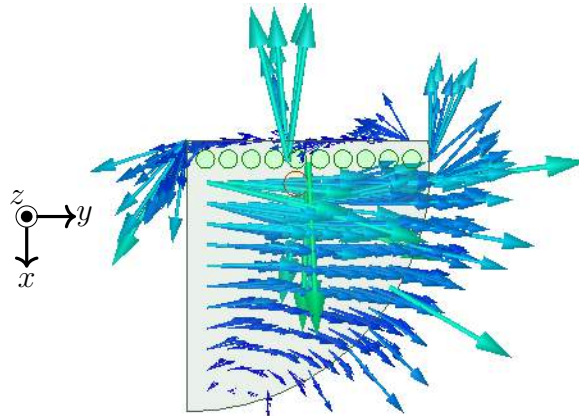
Figura 28 – Distribuição do campo magnético no interior da QCDRA com superfície de topo metálica.
