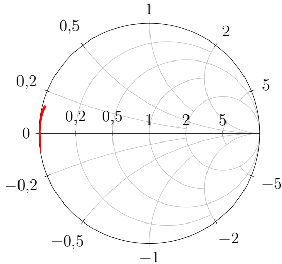
Figura 65 – Parâmetro S_{11} do toco radial simulado no HFSS.
