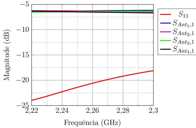
Figura 66 – Balanço de potência após inserção do conector SMA.
