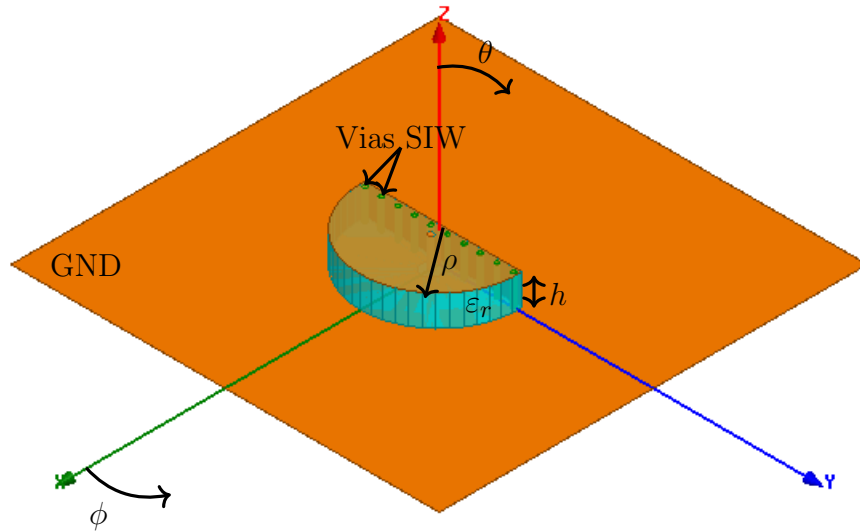
Figura 24 – Geometria reduzida para meio cilindro com superfície de topo metálica.
