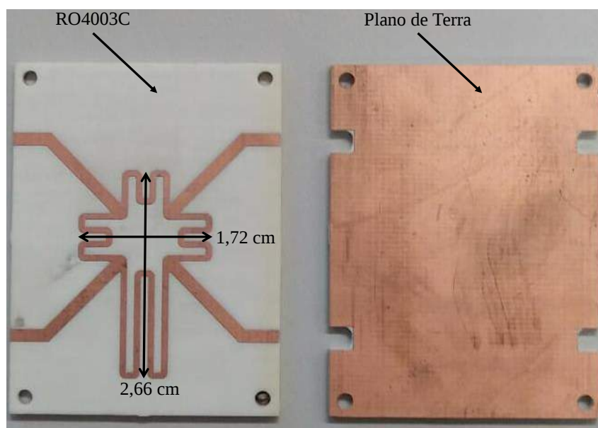
Figura 57 – Leiaute prototipado da híbrida de 180° em fresa.
