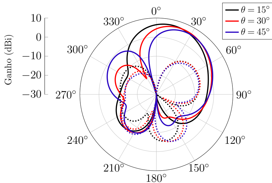
Figura 99 – Diagramas de irradiação com apontamento de feixe da rede 2 \times 2 em Banda L no plano \phi = 0^\circ . Linhas contínuas: Ganho RHCP. Linhas pontilhadas: Ganho LHCP.
