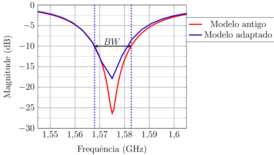
Figura 109 – Comparação entre os coeficientes de reflexão em função da frequência para a antena projetada em Banda L.
