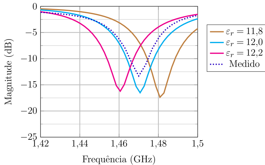
Figura 113 – Comparação entre o coeficiente de reflexão medido com coeficiente de reflexão simulado para diferentes valores de \epsilon_r .
