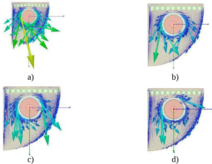
Figura 40 – Densidade de corrente superficial. a) Indutor em \phi = 0^\circ . b) Indutor em \phi = 45^\circ . c) Indutor em \phi = 90^\circ . d) Indutor em \phi = 135^\circ
