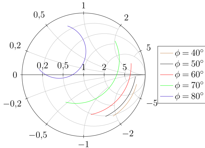
Figura 86 – Análise da impedância de entrada com a ponta de prova coaxial em \rho = 6 mm.
