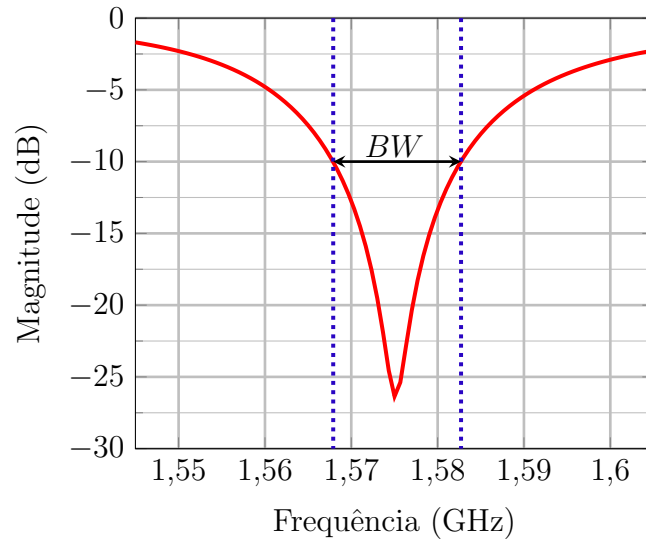
Figura 95 – Coeficiente de reflexão em função da frequência para a antena projetada em Banda L com indutor de 6,6 nH.
