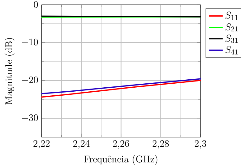
Figura 50 – Parâmetros S da híbrida de 90^\circ em stripline simulados.
