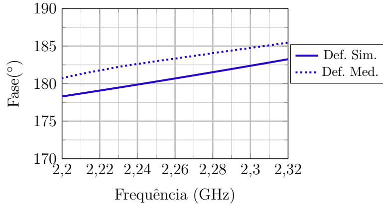
Figura 62 – Comparação dos resultados de defasagem relativa entre as portas 2 e 3 simulados e medidos.
