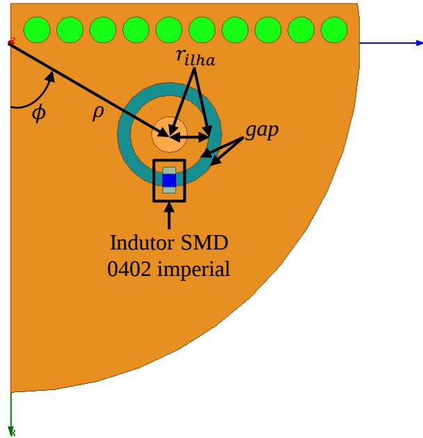
Figura 36 – QDCRA em Banda S com indutor na superfície de topo metálica.
