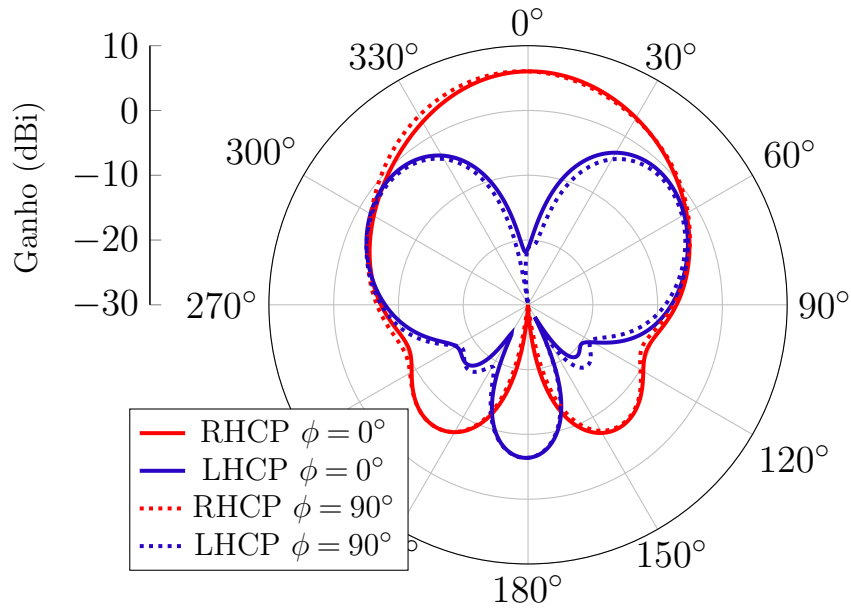
Figura 82 – Ganho RHCP e LHCP da rede 2×2 em Banda S com plano de terra do CubeSat 8U.
