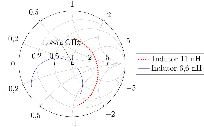
Figura 94 – Análise da impedância de entrada para r_{ilha} = 4 mm.
