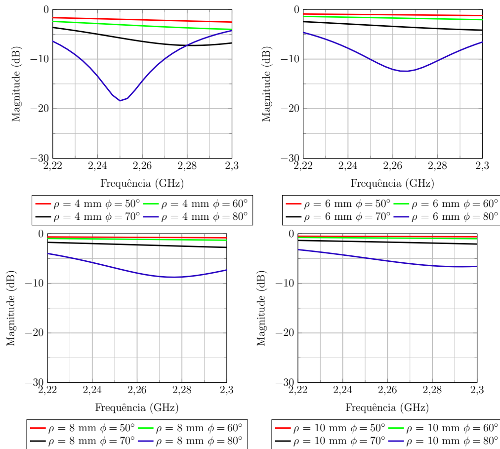
Figura 29 – Coeficientes de reflexão em função da frequência para diferentes posicionamentos da ponta de prova coaxial na QCDRA com superfície metálica.
