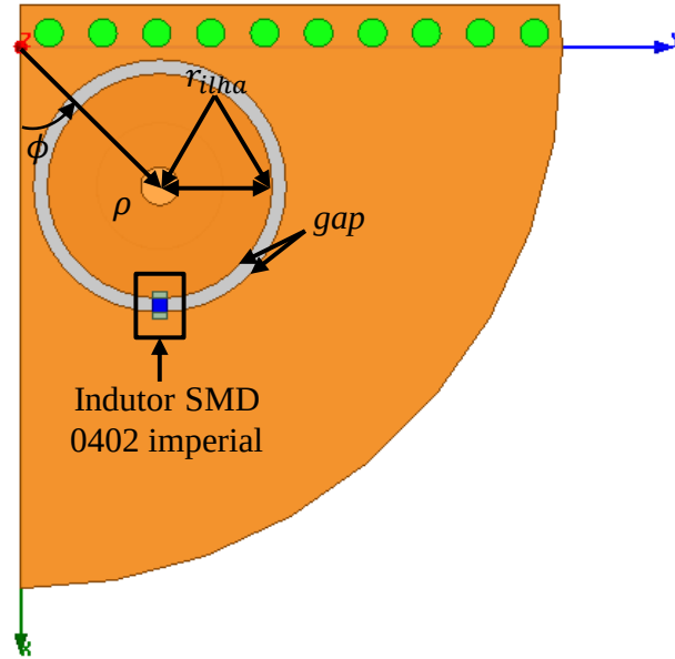
Figura 93 – Vista superior da QCDRA em Banda L com r_{ilha} = 4 mm.
