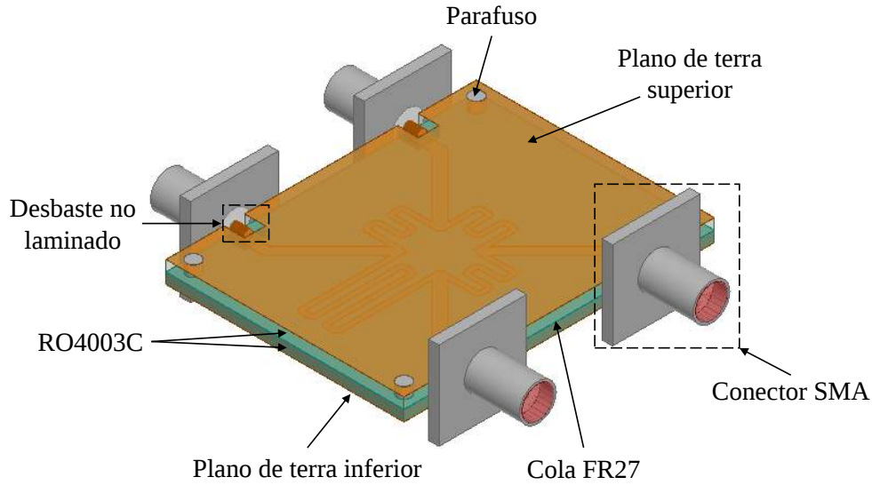
Figura 54 – Geometria completa da híbrida de 180° simulada no HFSS.
