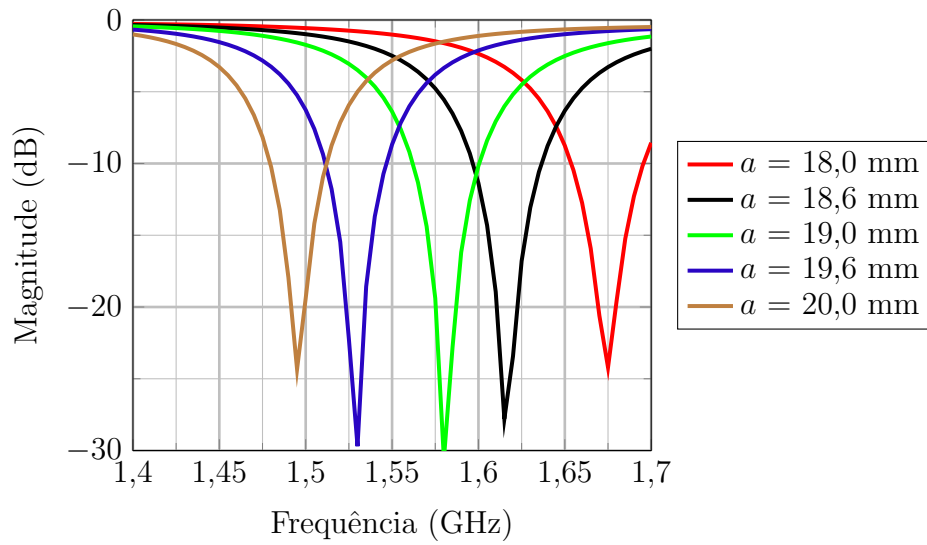
Figura 21 – Influência da variação do raio no coeficiente de reflexão em função da frequência para CDRA com superfície metálica.
