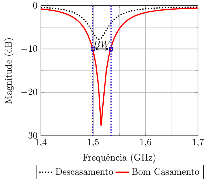
Figura 1 – Exemplo da curva de casamento de impedância.
