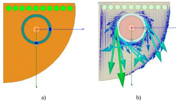
Figura 41 – DRA em Banda S com 2 indutores na superfície de topo metálica. a) Geometria. b) Distribuição de corrente.
