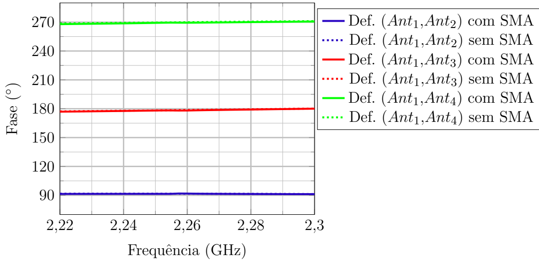
Figura 70 – Defasagem relativa após inserção do conector SMA.
