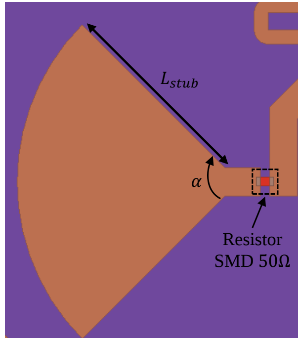
Figura 64 – Geometria clássica de um toco radial.
