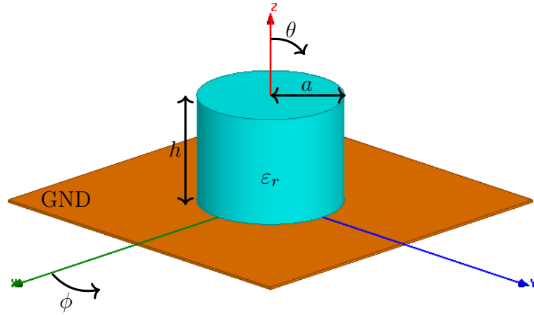
Figura 4 – Antena dielétrica ressoadora cilíndrica.
