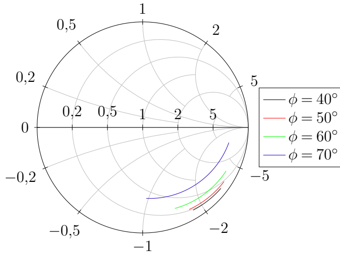
Figura 32 – Análise da impedância de entrada com a ponta de prova coaxial em \rho = 7 mm.
