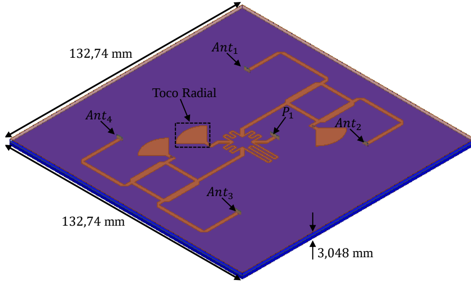
Figura 63 – Modelo eletromagnético do sistema alimentador completo.
