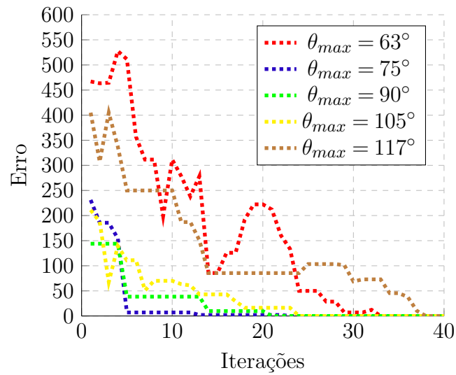
Figura 18 – Evolução do valor da função fitness para o melhor indivíduo para os casos especificados na Tabela 5.
