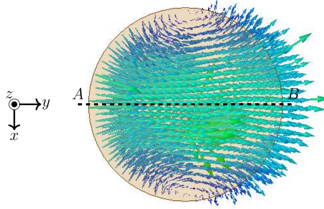
Figura 23 – Distribuição do campo magnético no interior da CDRA com superfície metálica.
