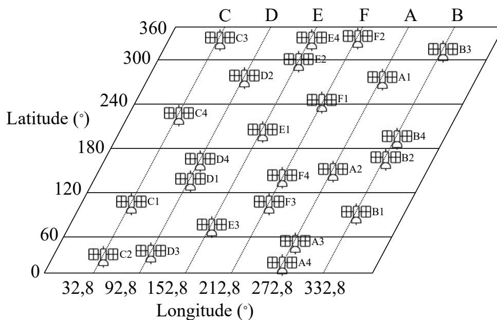
Figura 7 – Esquemático da constelação de satélites do sistema GPS.
