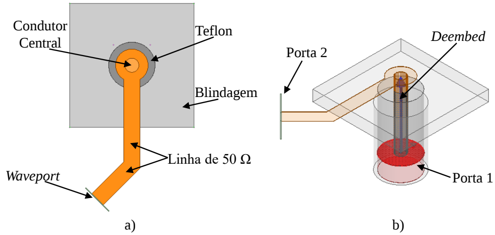
Figura 71 – Análise da transição entre SMA e Linha.
