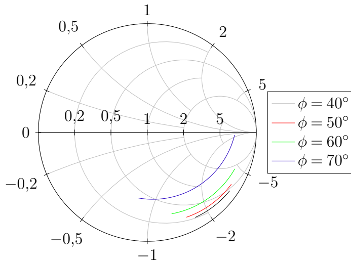
Figura 31 – Análise da impedância de entrada com a ponta de prova coaxial em \rho = 6 mm.
