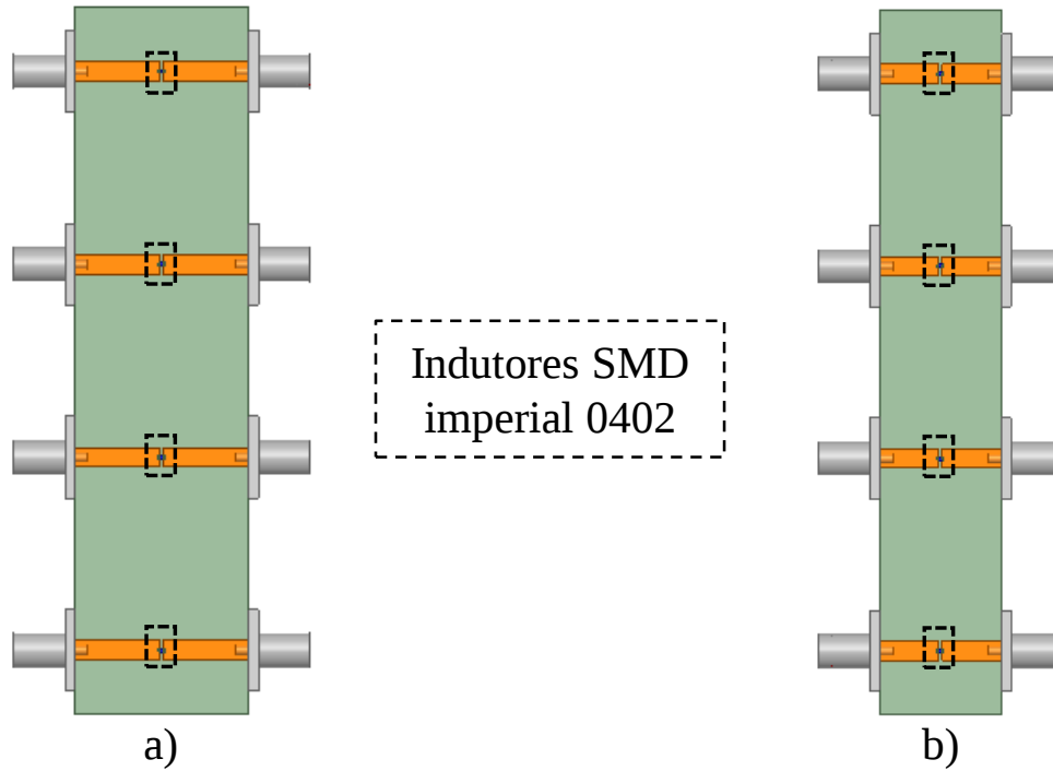
Figura 103 – Kits para teste de indutores. a) Geometria para 1,575 GHz. b) Geometria para 2,26 GHz.
