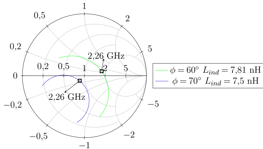
Figura 37 – Análise da impedância de entrada com a ponta de prova coaxial em \rho = 7 \, \text{mm} e com indutor na superfície de topo metálica.
