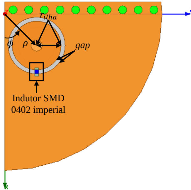
Figura 91 – Vista superior da QCDRA em Banda L com r_{ilha} = 3 mm.
