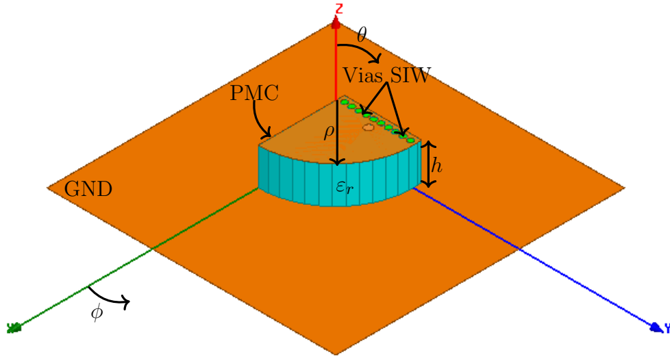
Figura 27 – Geometria reduzida para um quarto de cilindro com superfície de topo metálica.
