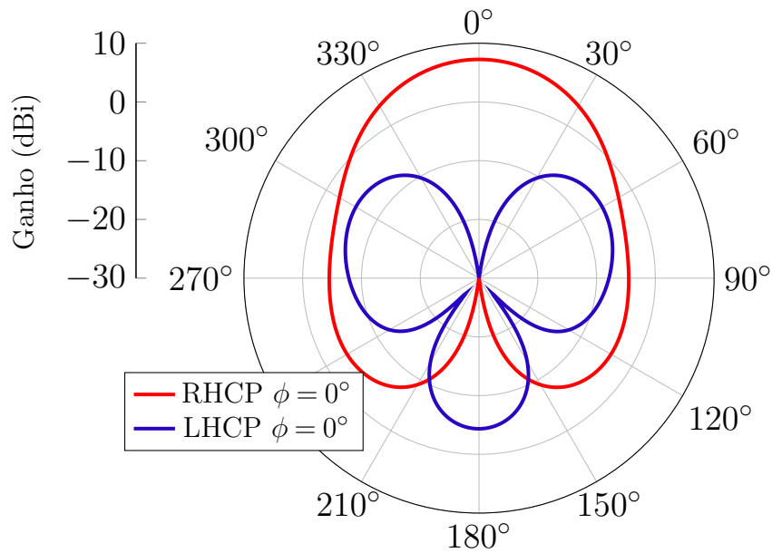
Figura 45 – Ganho RHCP e LHCP da rede 2×2 em Banda S com elementos em rotação sequencial.
