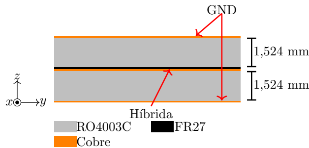
Figura 55 – Vista transversal da híbrida de 180° em stripline .
