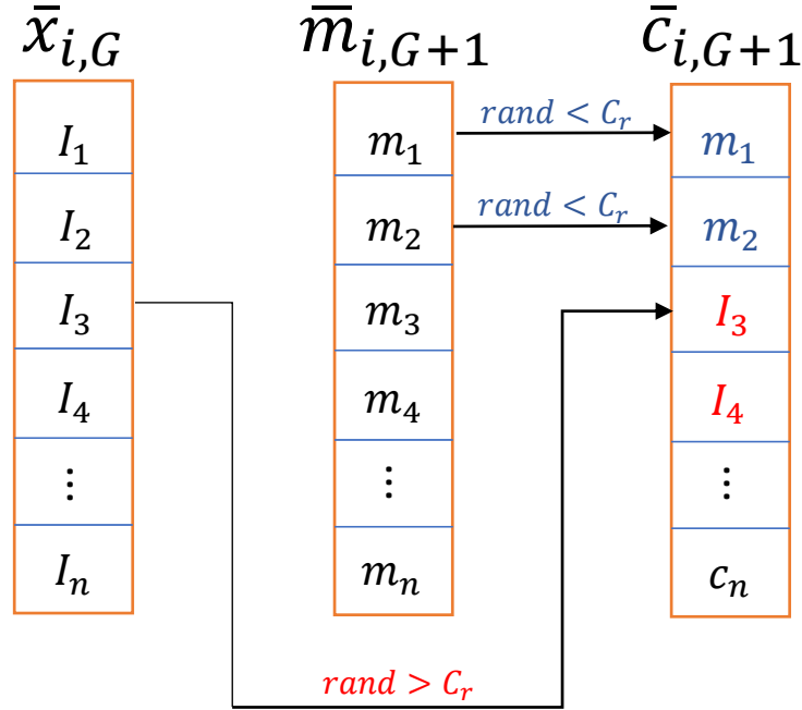
Figura 13 – Processo de crossover exponencial.
