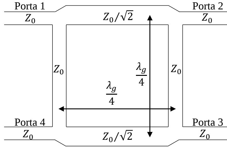
Figura 48 – Geometria da híbrida de 90°.
