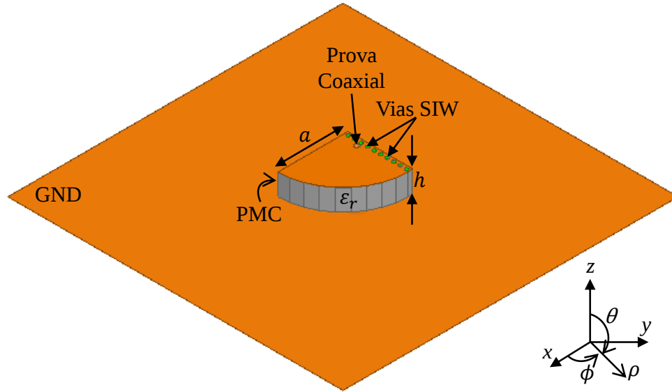
Figura 84 – Vista isométrica da DRA para Banda L.
