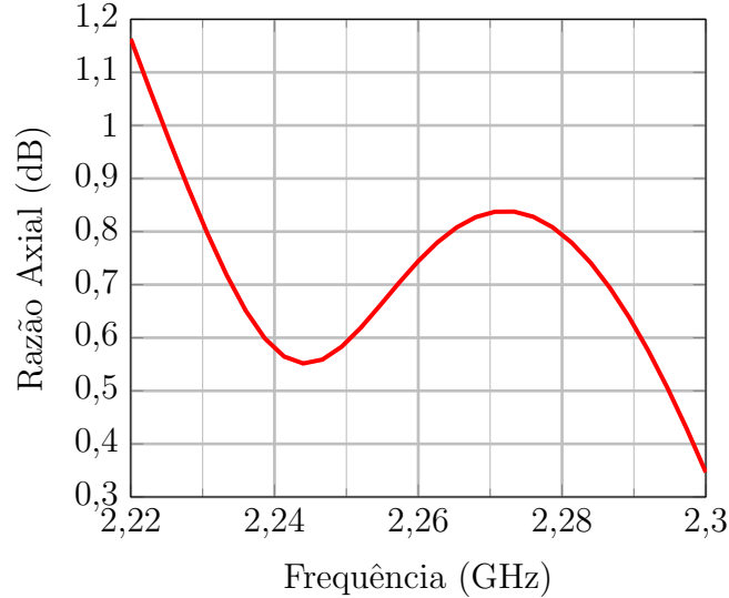
Figura 83 – Razão axial da rede 2×2 em Banda S com plano de terra do CubeSat 8U.
