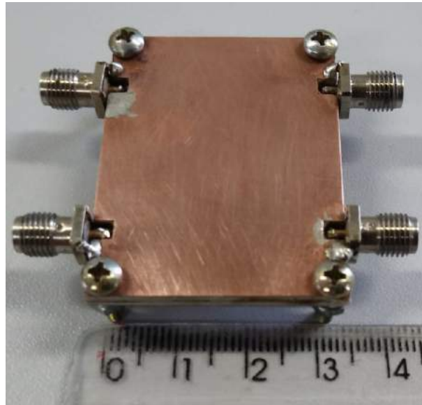
Figura 60 – Protótipo da híbrida de 180° construído.
