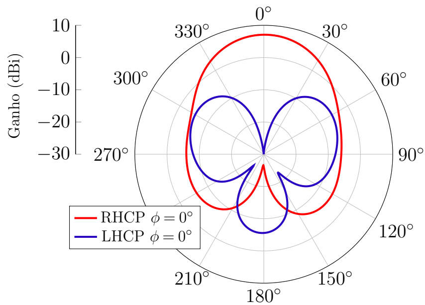
Figura 79 – Ganho RHCP e LHCP da rede 2×2 em Banda S com sistema de alimentação integrado.
