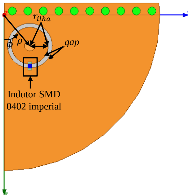
Figura 88 – Vista superior da QCDRA em Banda L com indutor.
