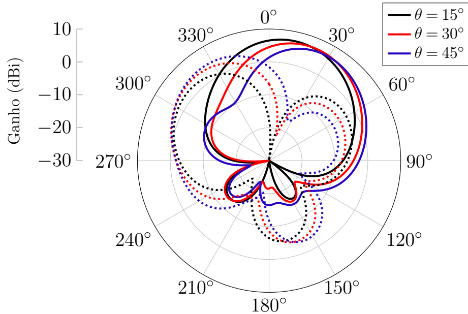
Figura 100 – Diagramas de irradiação com apontamento de feixe da rede 2 \times 2 em Banda L no plano \phi = 45^\circ . Linhas contínuas: Ganho RHCP. Linhas pontilhadas: Ganho LHCP.
