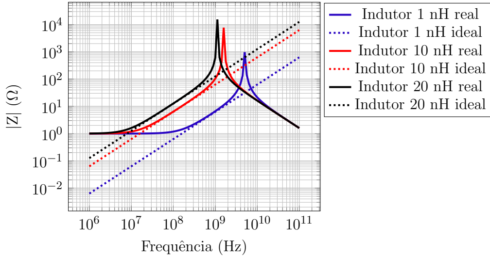
Figura 35 – Análise da frequência de ressonância própria de um indutor.
