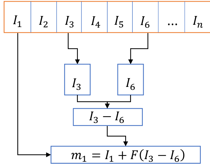
Figura 11 – Processo de mutação.
