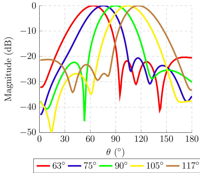
Figura 17 – Diagramas de irradiação obtidos com os coeficientes de excitação otimizados para os casos especificados na Tabela 5.
