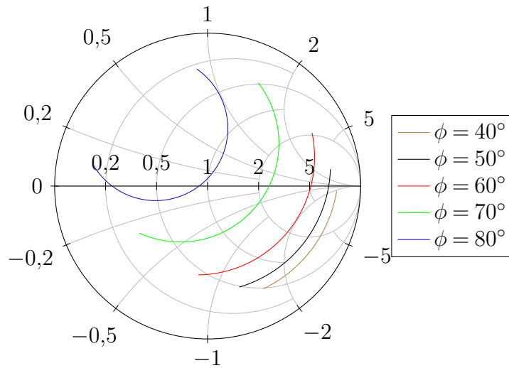
Figura 85 – Análise da impedância de entrada com a ponta de prova coaxial em \rho = 5 mm.
