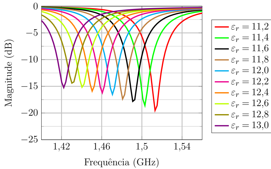
Figura 112 – Coeficiente de reflexão em função da frequência variando-se a constante dielétrica do material.
