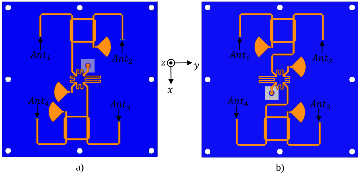
Figura 75 – Sistema de alimentação com parafusos. a) geometria sem modificação. b) geometria modificada para garantir polarização RHCP.
