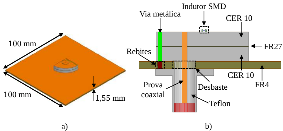
Figura 108 – Modelo adaptado da antena projetada em Banda L. a) Vista isométrica. b) Vista corte lateral.
