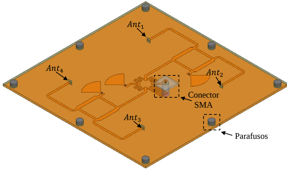
Figura 73 – Sistema de alimentação com parafusos ao redor da estrutura.
