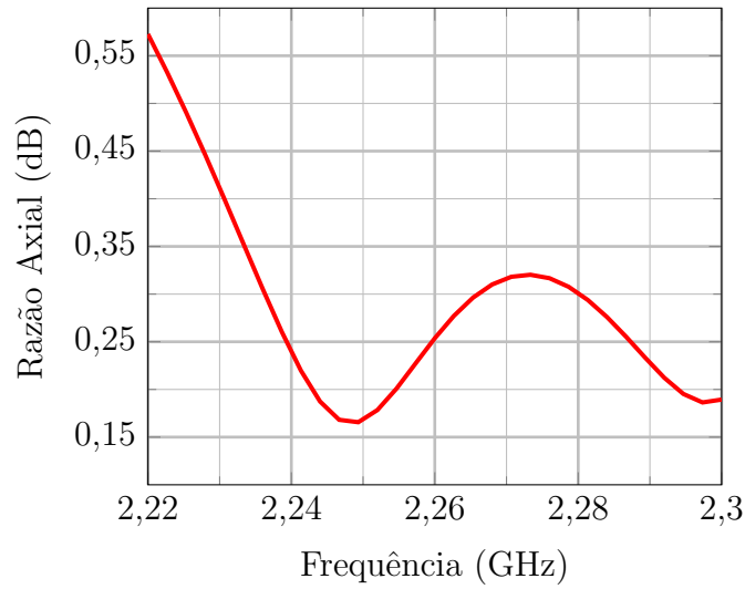
Figura 80 – Razão axial da rede 2×2 em Banda S com sistema de alimentação integrado.
