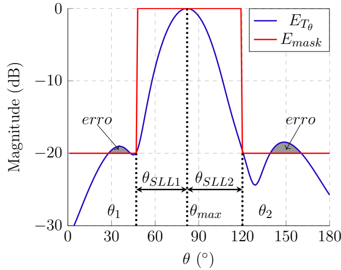
Figura 15 – Definições de máscara e diagrama de irradiação calculado para casos de apontamento de feixe e controle do nível dos lóbulos secundários.
