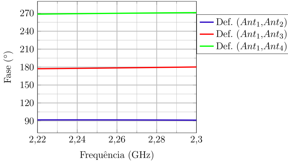
Figura 67 – Defasagem relativa do sistema de alimentação.
