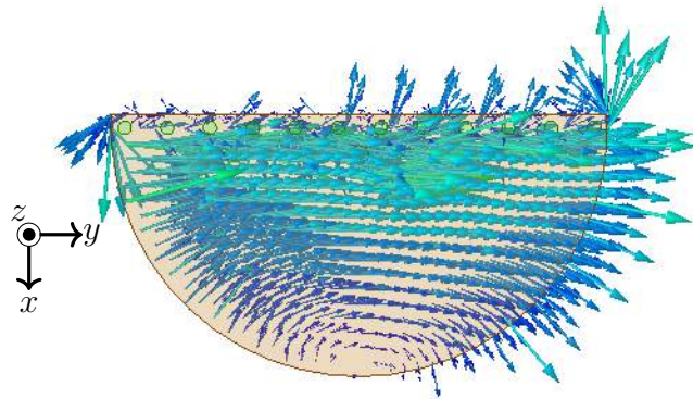
Figura 25 – Distribuição do campo magnético no interior da HCDRA com superfície de topo metálica.
