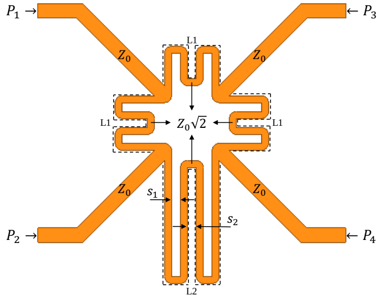
Figura 53 – Modelo da híbrida de 180° compacta projetada no HFSS.
