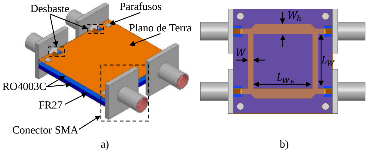
Figura 49 – Híbrida de 90^\circ projetada no HFSS. a) Vista isométrica. b) Vista superior.
