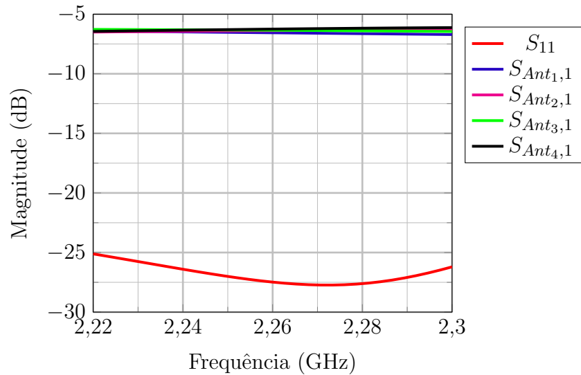
Figura 76 – Balanço de potência após modificação do sistema alimentador.
