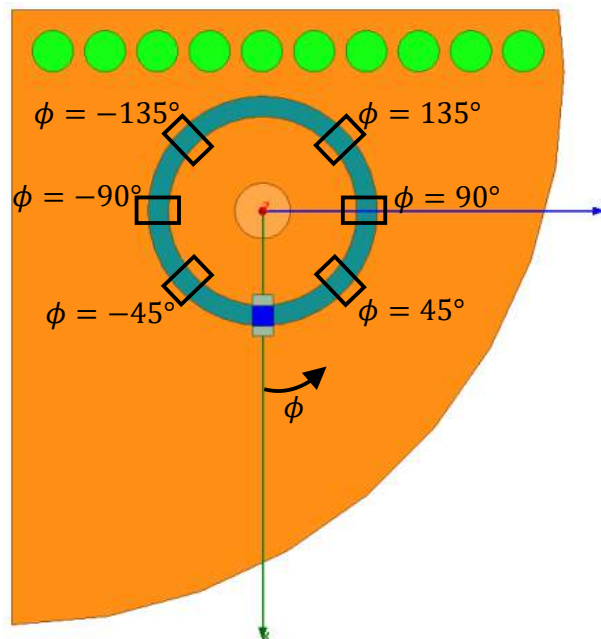
Figura 39 – Variação do posicionamento dos indutores na superfície de topo metálica.
