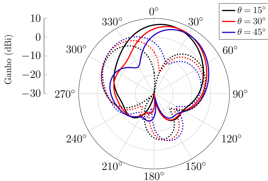
Figura 101 – Diagramas de irradiação com apontamento de feixe da rede 2 \times 2 em Banda L no plano \phi = 60^\circ . Linhas contínuas: Ganho RHCP. Linhas pontilhadas: Ganho LHCP.
