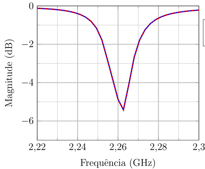
Figura 72 – Análise da transição entre conector SMA e linha.
