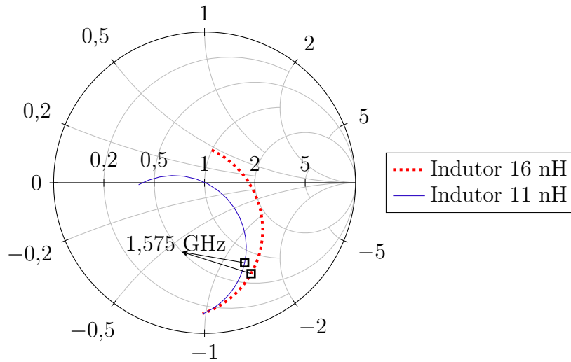
Figura 92 – Análise da impedância de entrada após inserção do indutor de 16 nH.
