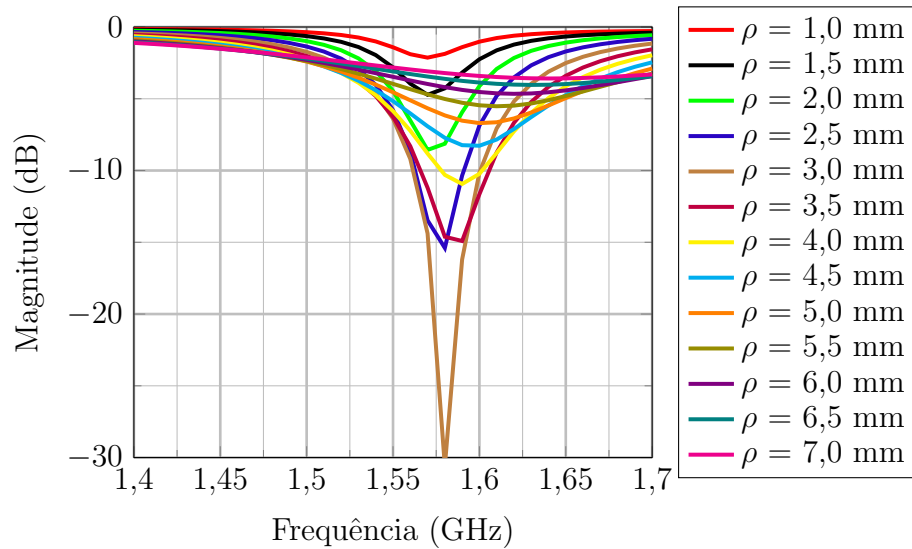
Figura 22 – Influência do posicionamento da ponta de prova coaxial no coeficiente de reflexão em função da frequência para CDRA com superfície metálica.
