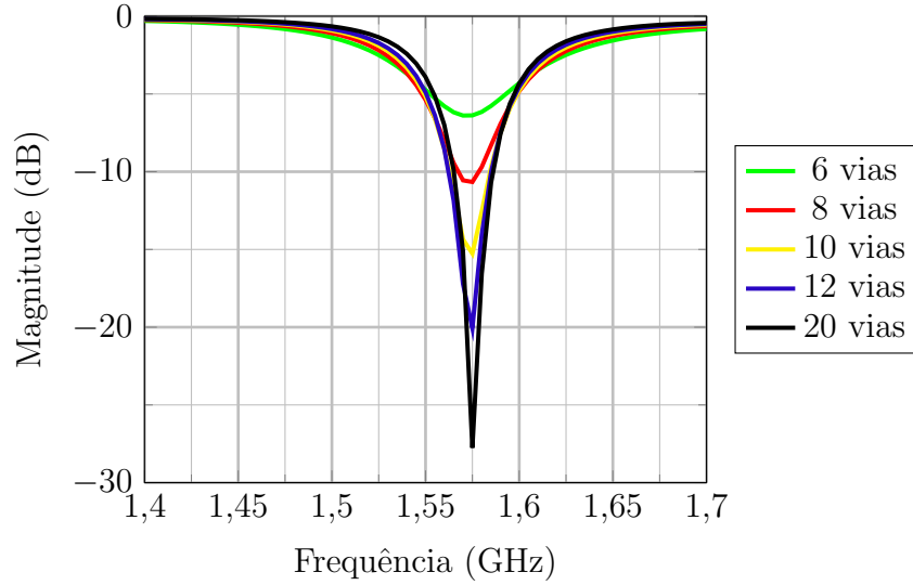
Figura 26 – Influência do número de vias SIW no coeficiente de reflexão em função da frequência para a HCDRA com superfície de topo metálica.
