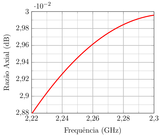
Figura 46 – Razão axial da rede 2×2 em Banda S com rotação sequencial.
