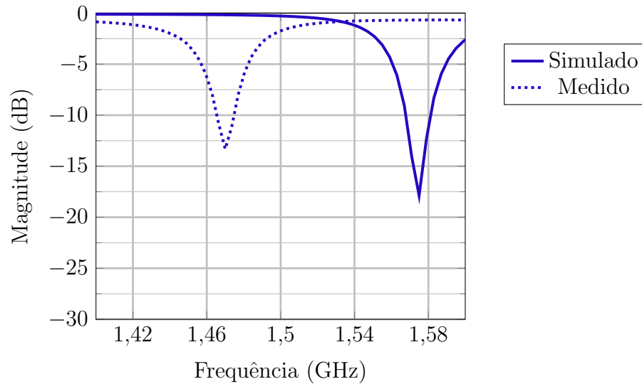
Figura 111 – Comparação entre o coeficiente de reflexão em função da frequência para a antena projetada em Banda L utilizando FR4 como plano de terra.
