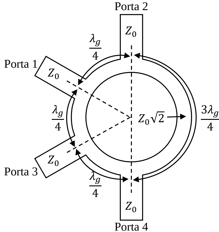
Figura 52 – Geometria convencional da híbrida de 180°.
