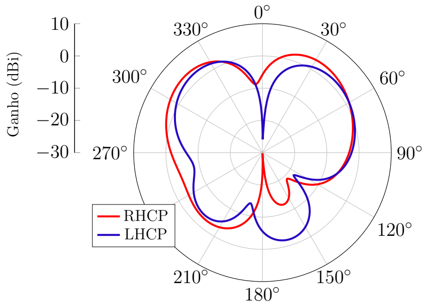
Figura 43 – Ganho RHCP e LHCP da rede 2 \times 2 em Banda S.
