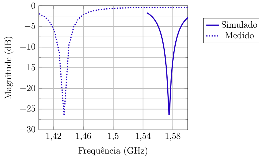
Figura 107 – Comparação entre o coeficiente de reflexão em função da frequência para a antena projetada em Banda L.
