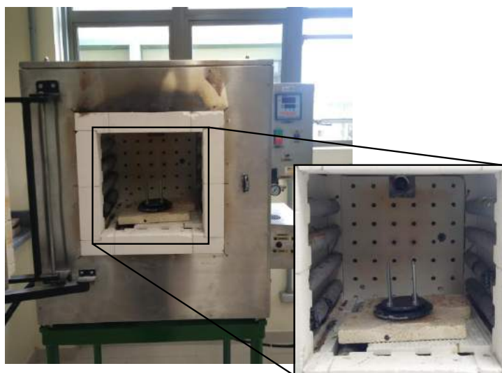
Figura 59 – Protótipo no interior da mufla.
