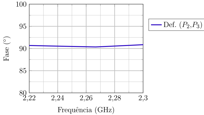
Figura 51 – Defasagem relativa entre as portas 2 e 3.
