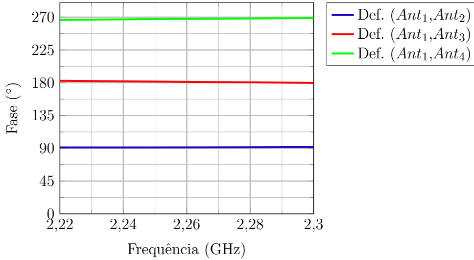
Figura 77 – Defasagem relativa após modificação do sistema de alimentação.
