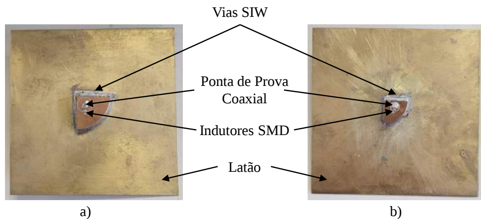
Figura 106 – Primeiros protótipos construídos. a) Banda L. b) Banda S.
