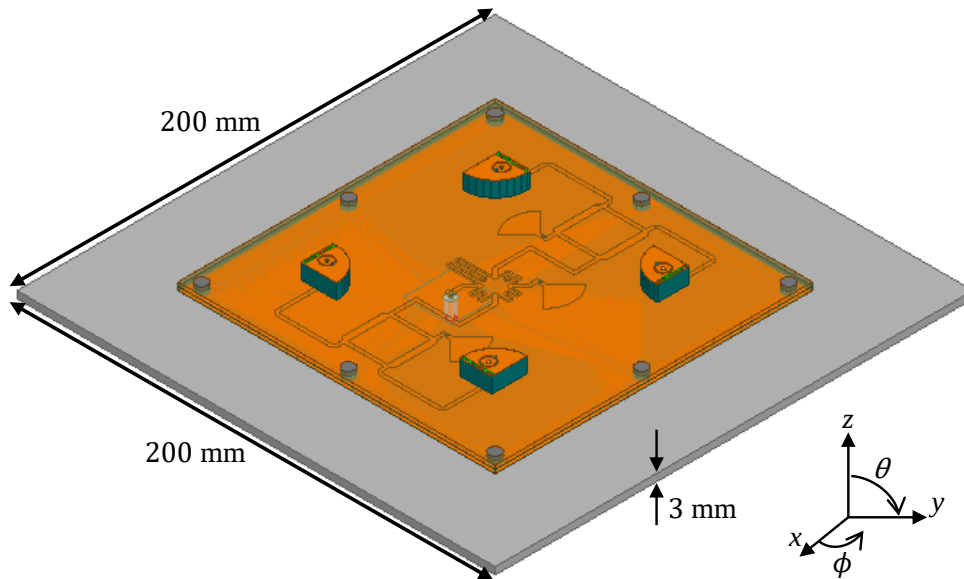
Figura 81 – Modelo eletromagnético da rede planar 2×2 em Banda S com plano de terra do CubeSat 8U.
