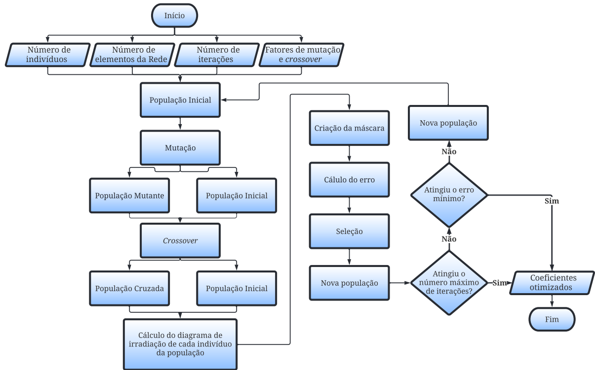
Figura 16 – Fluxograma do algoritmo Differential Evolution para otimização da rede de antenas.
