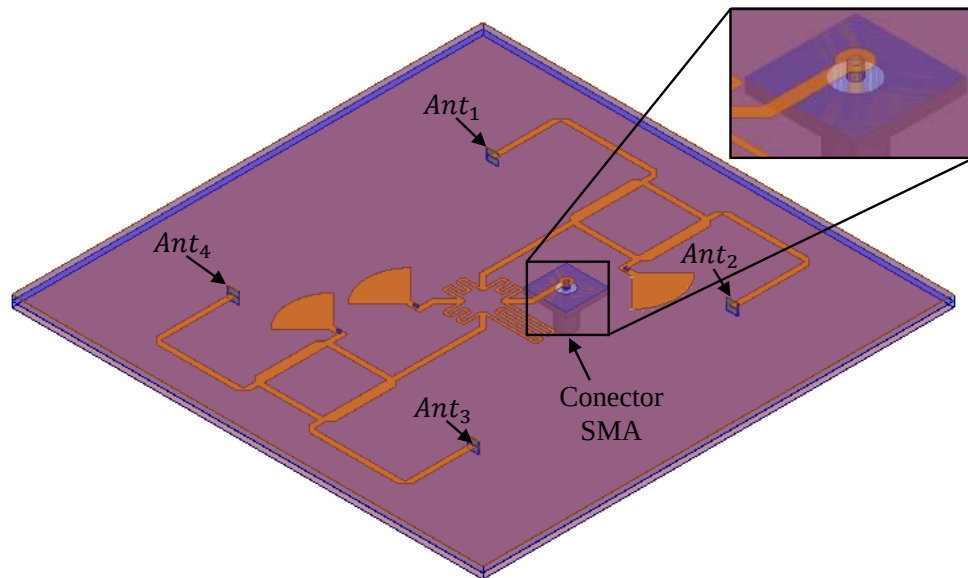
Figura 68 – Sistema de alimentação com conector SMA.
