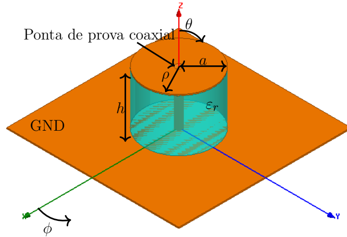
Figura 20 – CDRA-CM com excitação através de uma ponta de prova coaxial.
