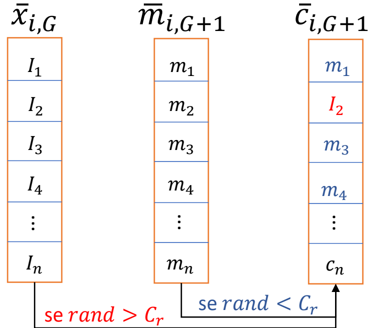
Figura 12 – Processo de crossover binomial.
