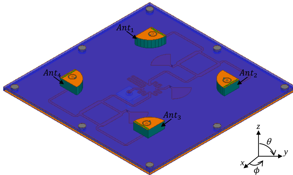
Figura 78 – Modelo eletromagnético da rede planar 2×2 em Banda S com o sistema de alimentação.
