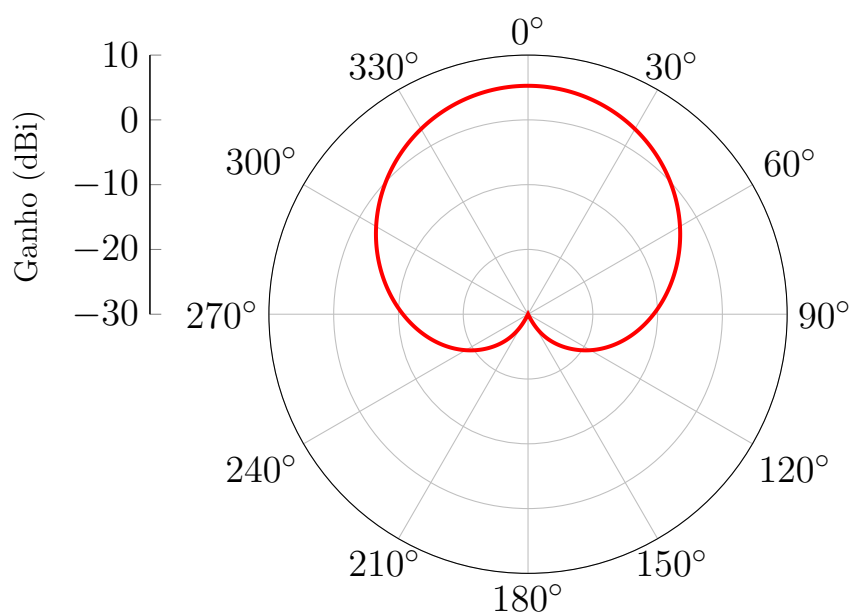
Figura 9 – Diagrama de irradiação broadside de uma rede de antenas 2x2 com rotação sequencial para operação em Banda L.
