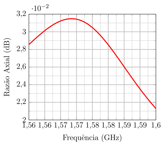
Figura 98 – Razão axial da rede 2×2 em Banda L com elementos dispostos em rotação sequencial.
