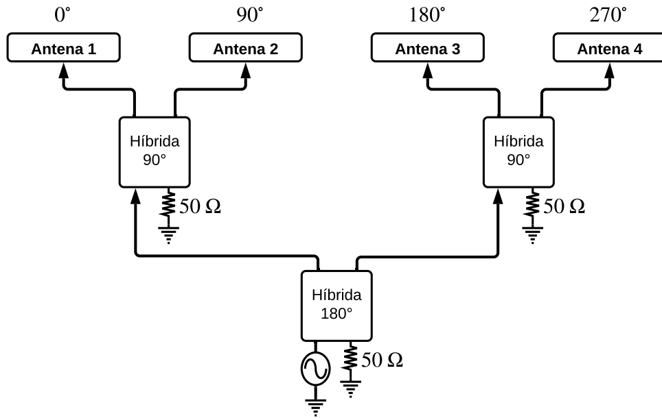
Figura 47 – Esquemático do sistema de alimentação da rede 2×2 em Banda S.
