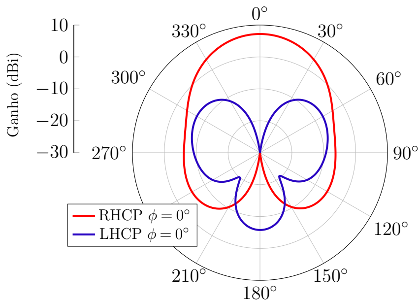
Figura 97 – Ganho RHCP e LHCP da rede 2×2 em Banda L com elementos dispostos em rotação sequencial.
