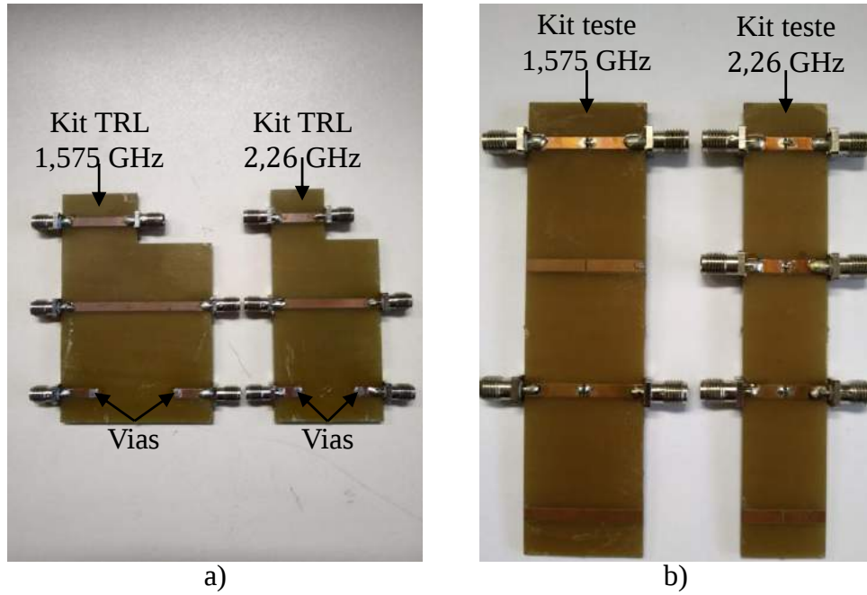
Figura 104 – Kits construídos a) TRL. b) Teste dos componentes.
