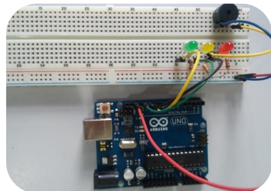
Circuito feito por alunos da Turma 80/ 8°
