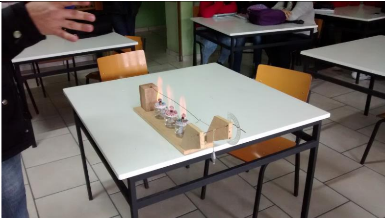
Dilatômetro linear
