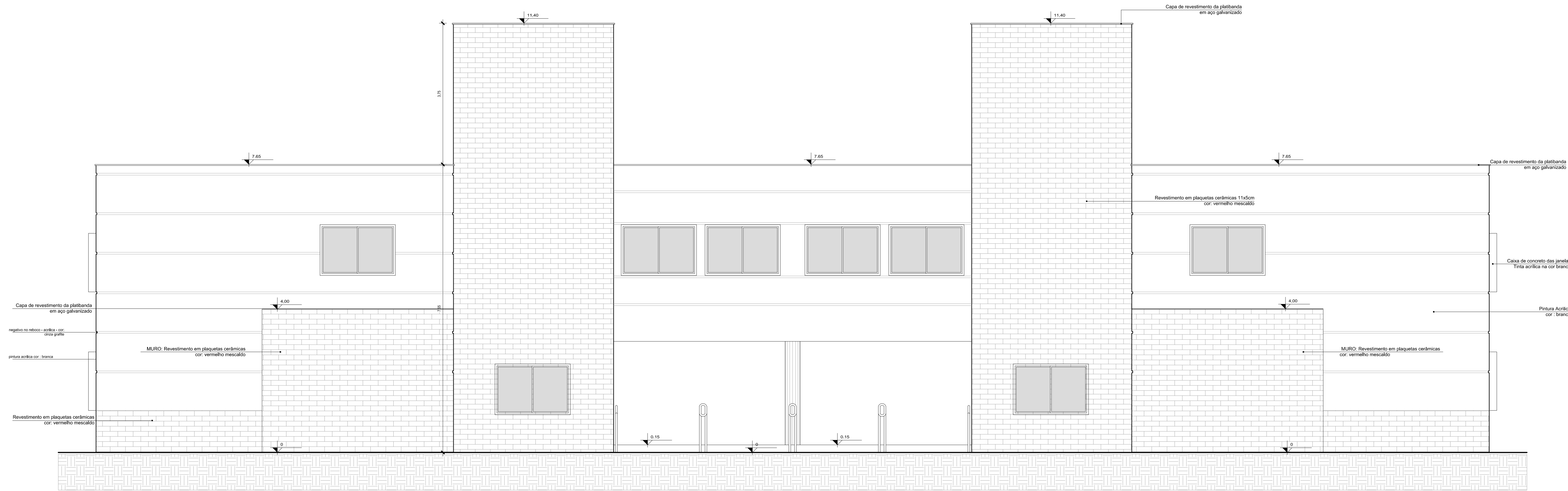
FACHADA 01 ESC: 1/50
