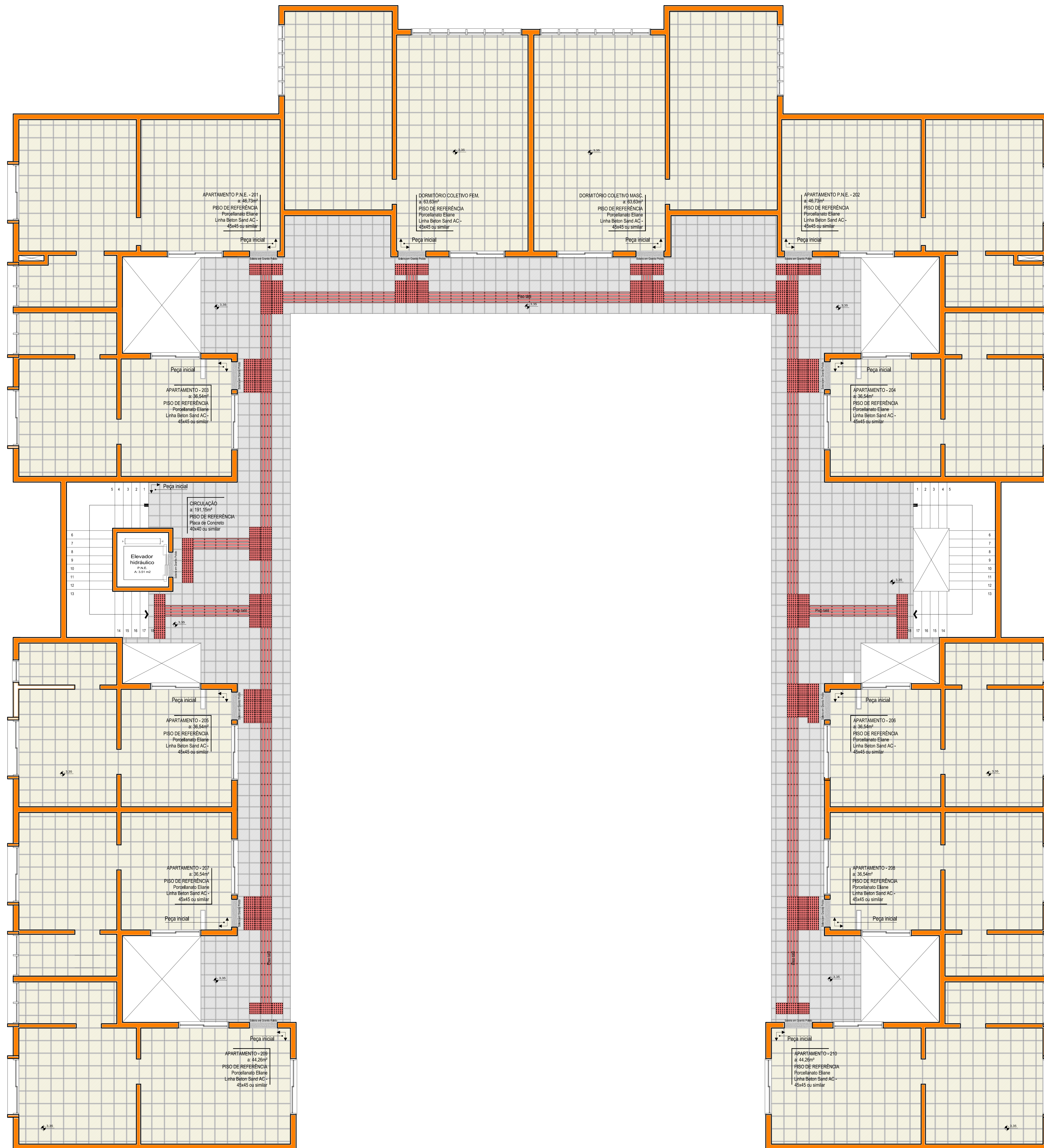
Planta de piso - 2º Pavimento Esc.:1/50 Área edificada: 899,55 m²
