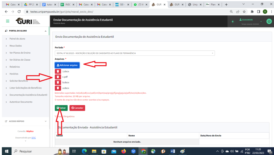
Figura 3: Adicionar Arquivos.
